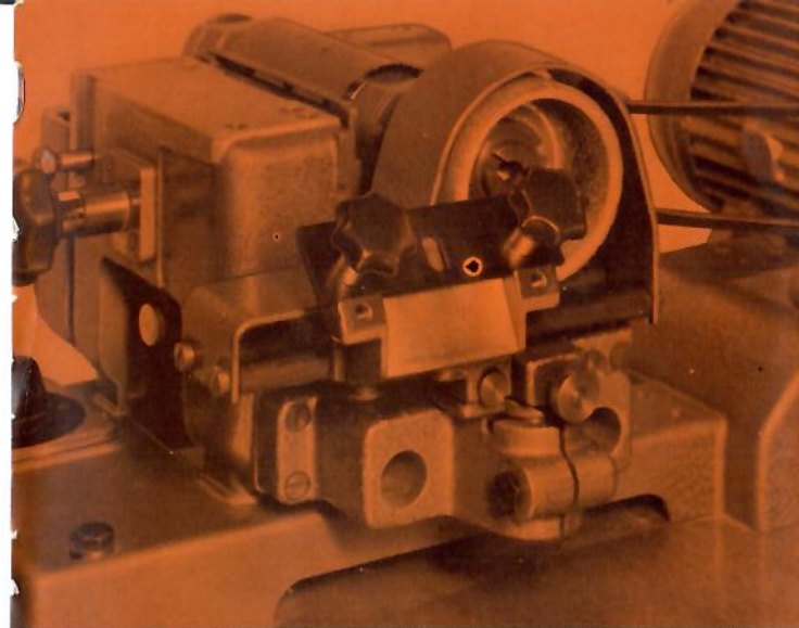
Schärfen eines Abrichthobelmessers mit der ULMIA universa-Schärfleinrichtung
