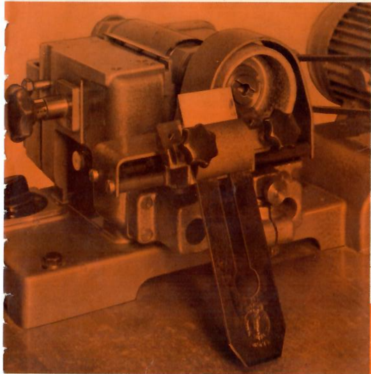
Schärfen eines Fasthobeleisens mit der ULMIA universa-Schärfleinrichtung
